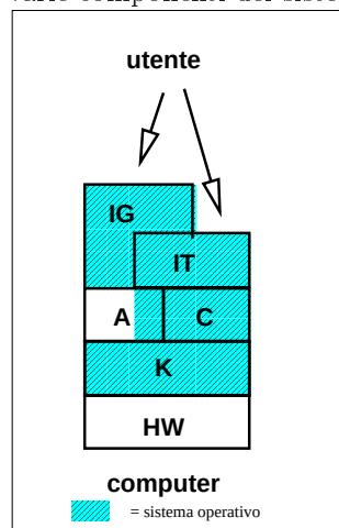
Figura 3.5: varie componenti del sistema operativo
