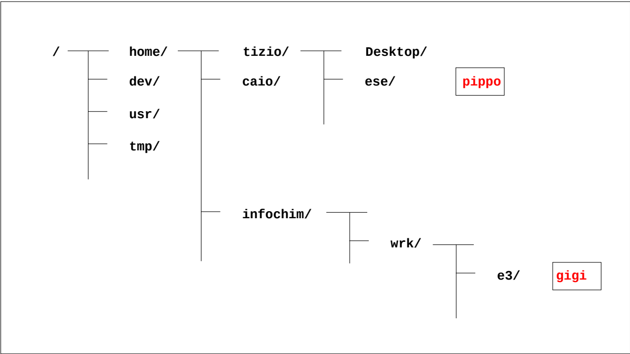
Figura 4.1: esempio di percorsi
